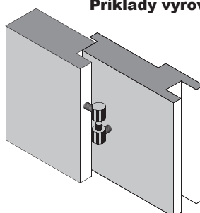
Příklady vyrovnaní dveří Příklady vyrovnanie dverí
